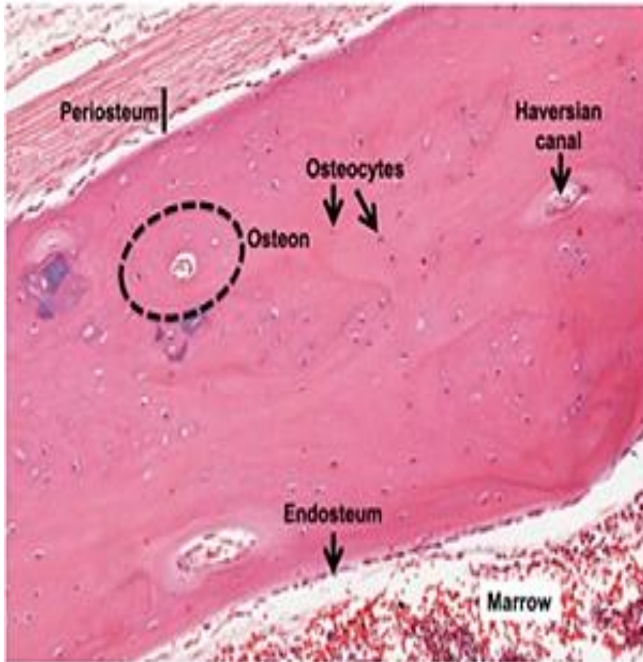
Compact bone
